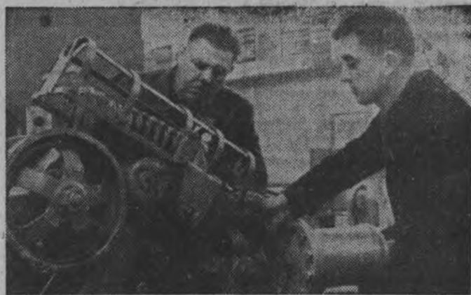
Москва. Стенд «ОПР-1402М» Тартуского ремзавода (Эстонская ССР) предназначен для разборки и сборки кареток подвески тракторов «ДТ-54», «ДТ-75», «Т-74». Его внедрение позволяет в полтора раза повысить производительность труда, дает значительную экономию. Эту новинку можно увидеть в ВДНХ СССР в экспозиции, которая знакомит с передовой технологией обслуживания машинно-тракторного парка.
